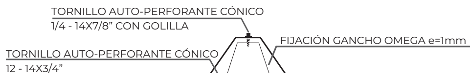
Fijación Gancho Omega
